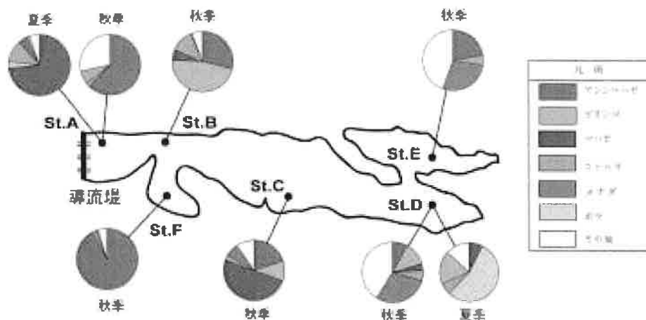
図 2-1-8 (1) 場所ごとの優占種個体数割合（平成 16 年（2004 年）夏季・秋季調査結果）（出典⑩）
